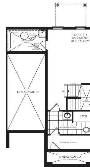
OPT. BASEMENT 'A' & 'B'
